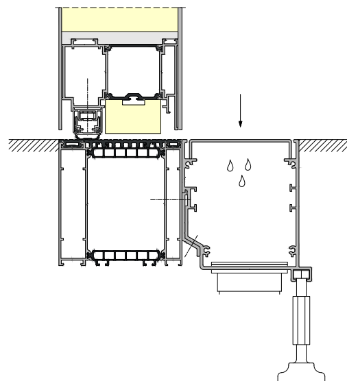
LINEARE ENTWÄSSERUNG IM RAHMEN DES SYSTEMS TM 102HI
