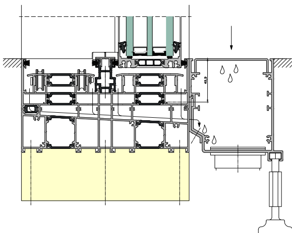
LINEARE ENTWÄSSERUNG IM RAHMEN DES SYSTEMS MOREVIEW
