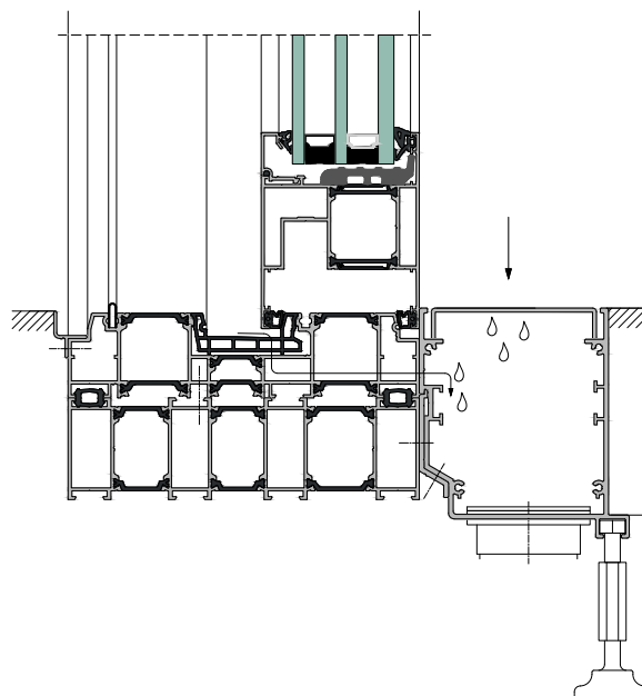
LINEARE ENTWÄSSERUNG IM RAHMEN DES SYSTEMS DP 180
